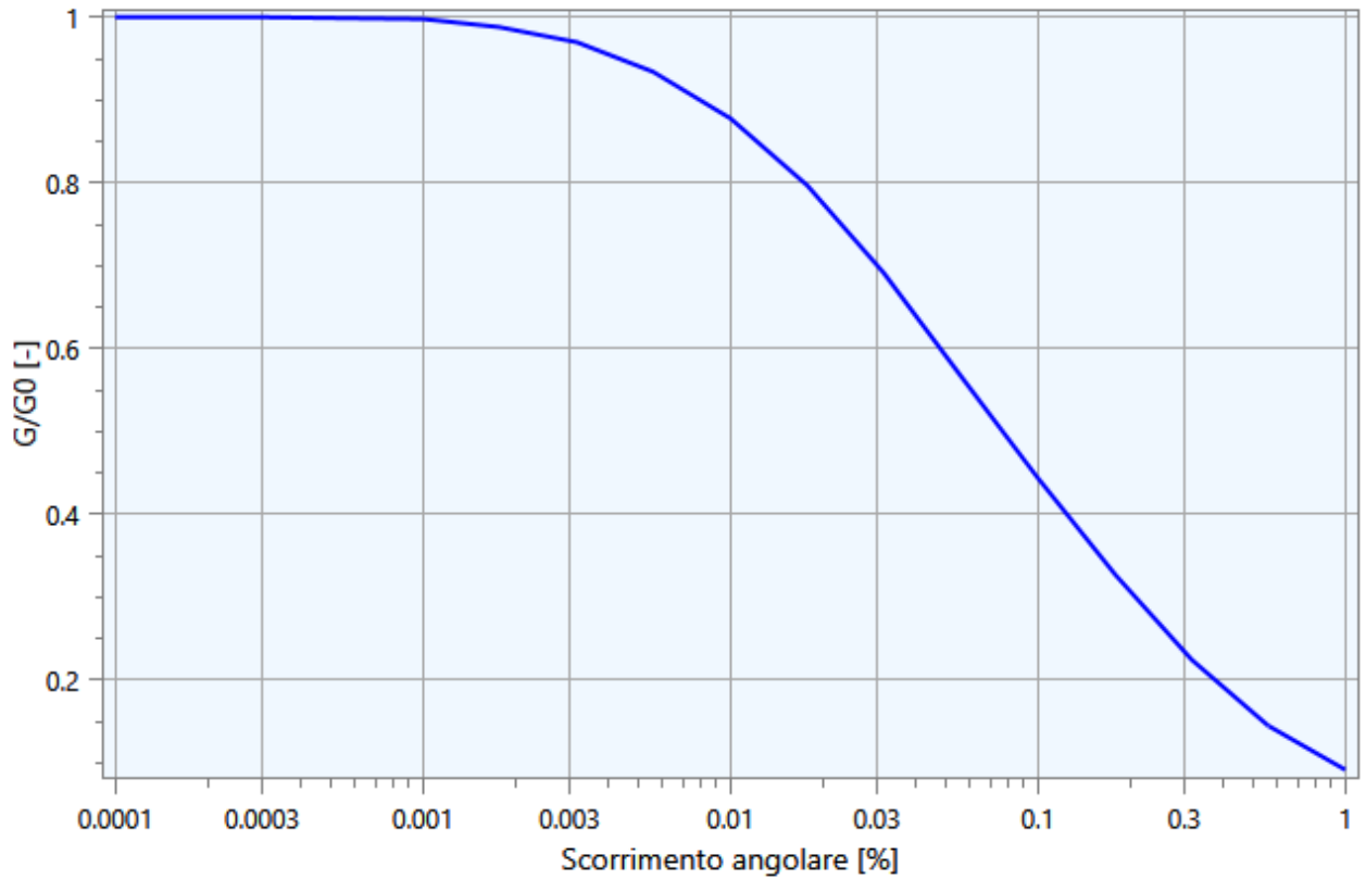
Modulo di taglio EPRI (93), 50-120 ft
