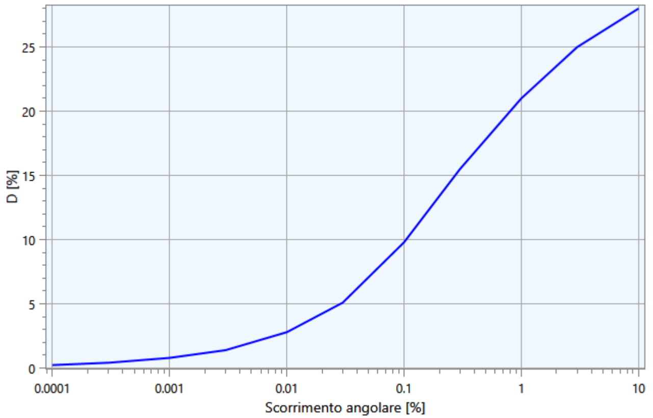
Smorzamento Sand Seed & Idriss (1970)
