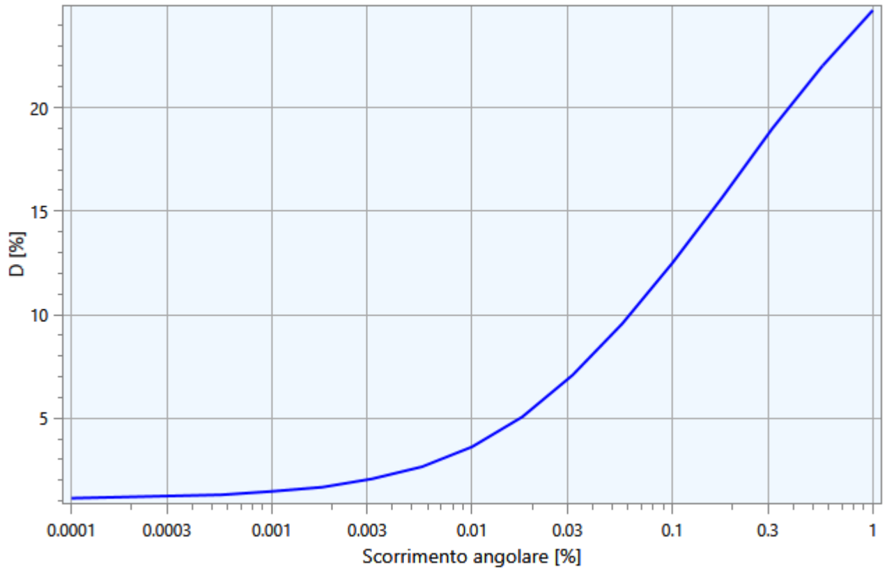
Smorzamento EPRI (93), 20-50 ft
