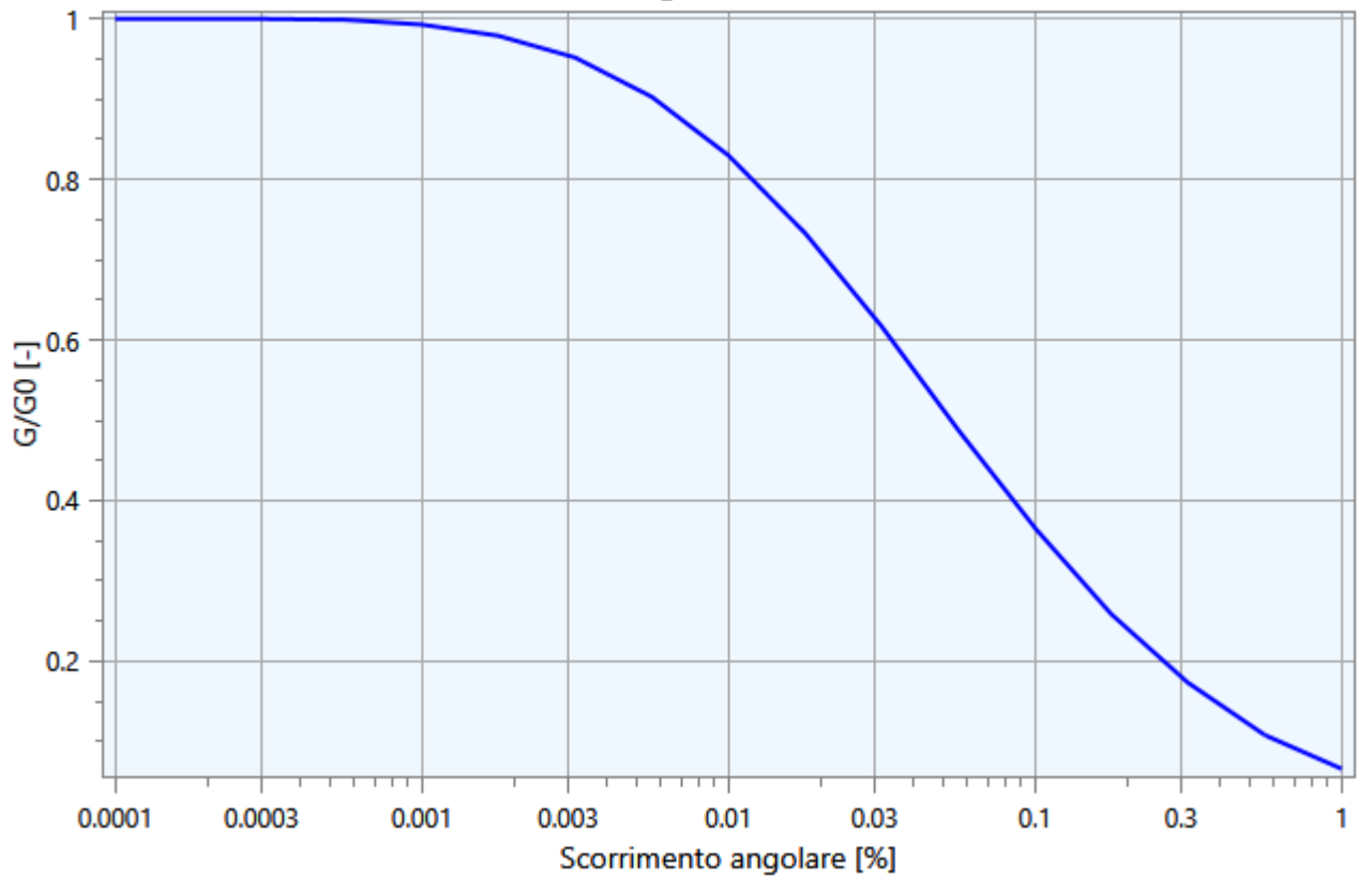
Modulo di taglio EPRI (93), 20-50 ft
