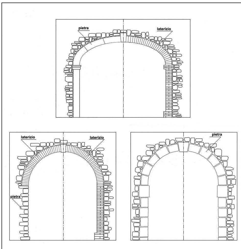
D.4.2 – Archi – Modelli tipologici edilizia tradizionale
