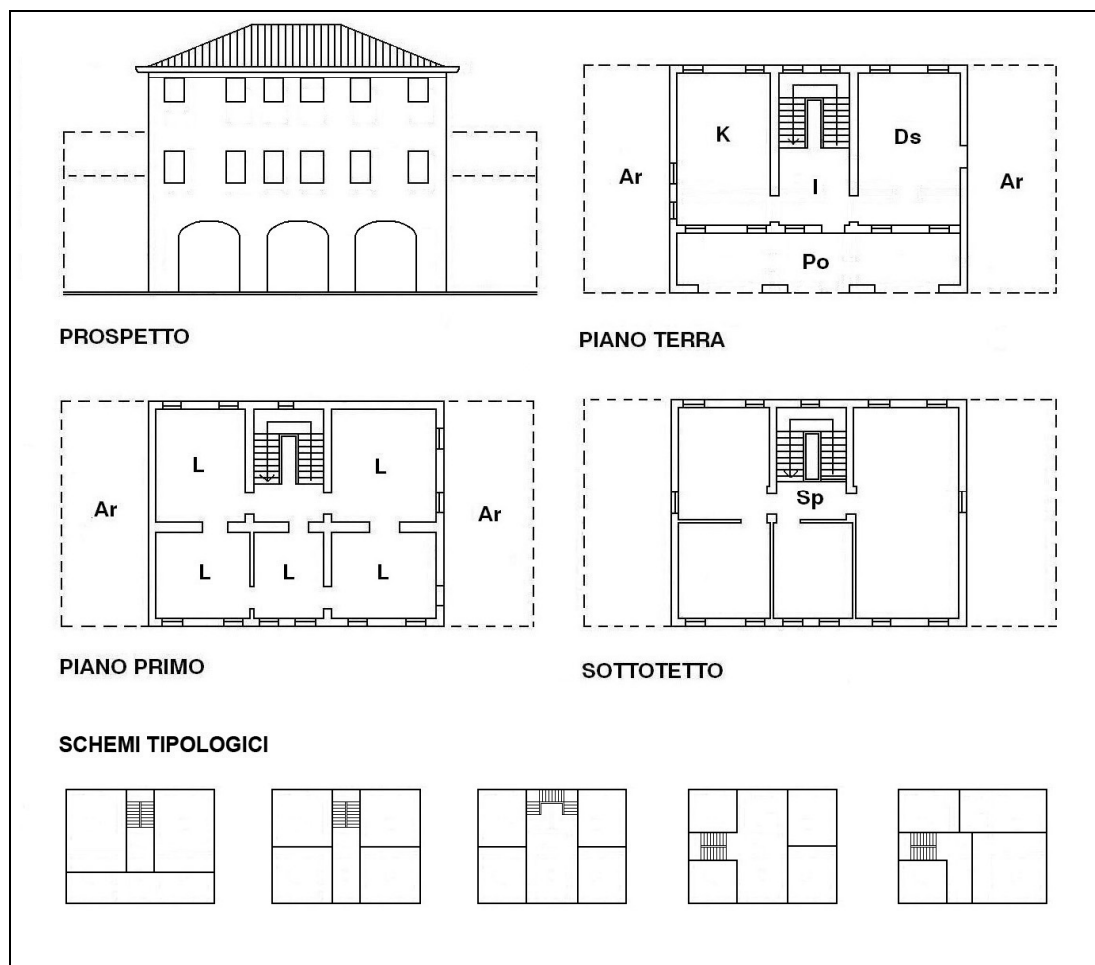
Tipologia con copertura a con portico – Schemi tipologici
