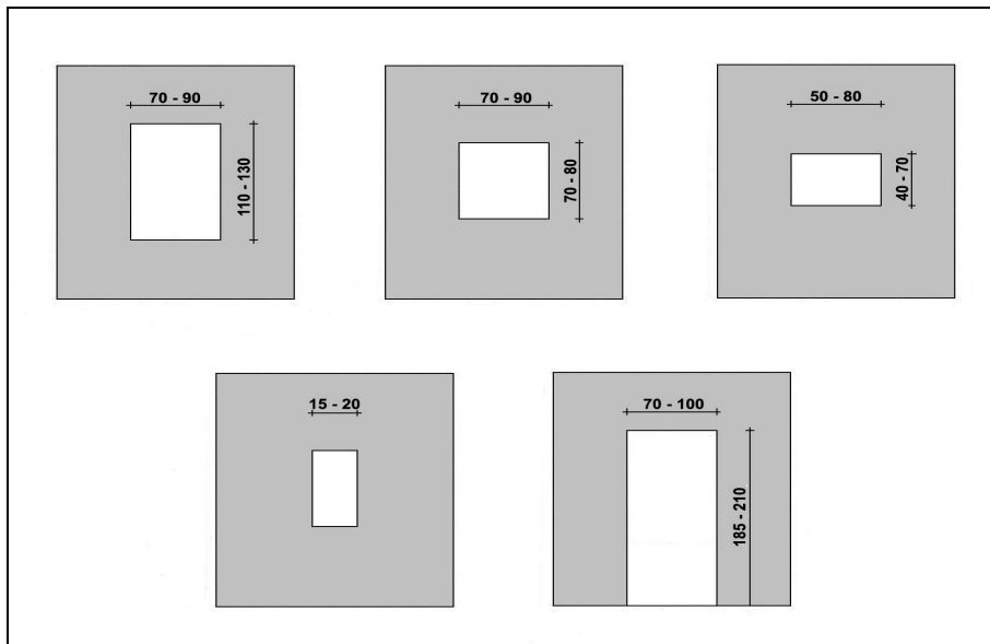
D.8 – Sottosistema aperture – Forometria abaco dimensionale
