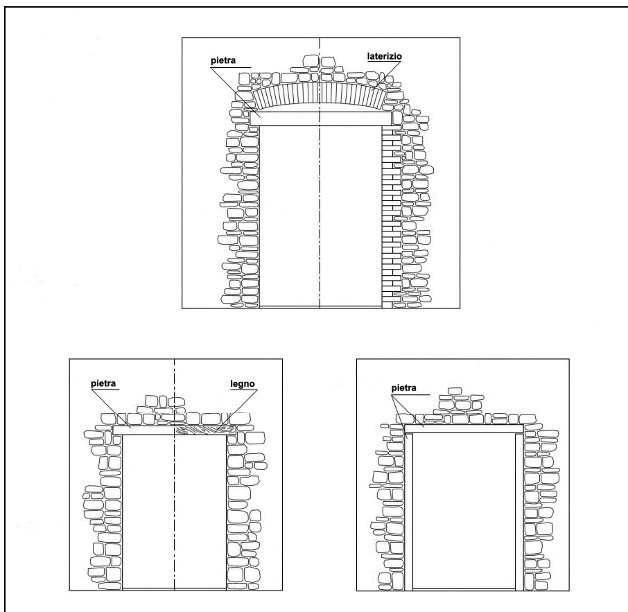
D.8.2 – Porte – Modelli tipologici edilizia tradizionale
