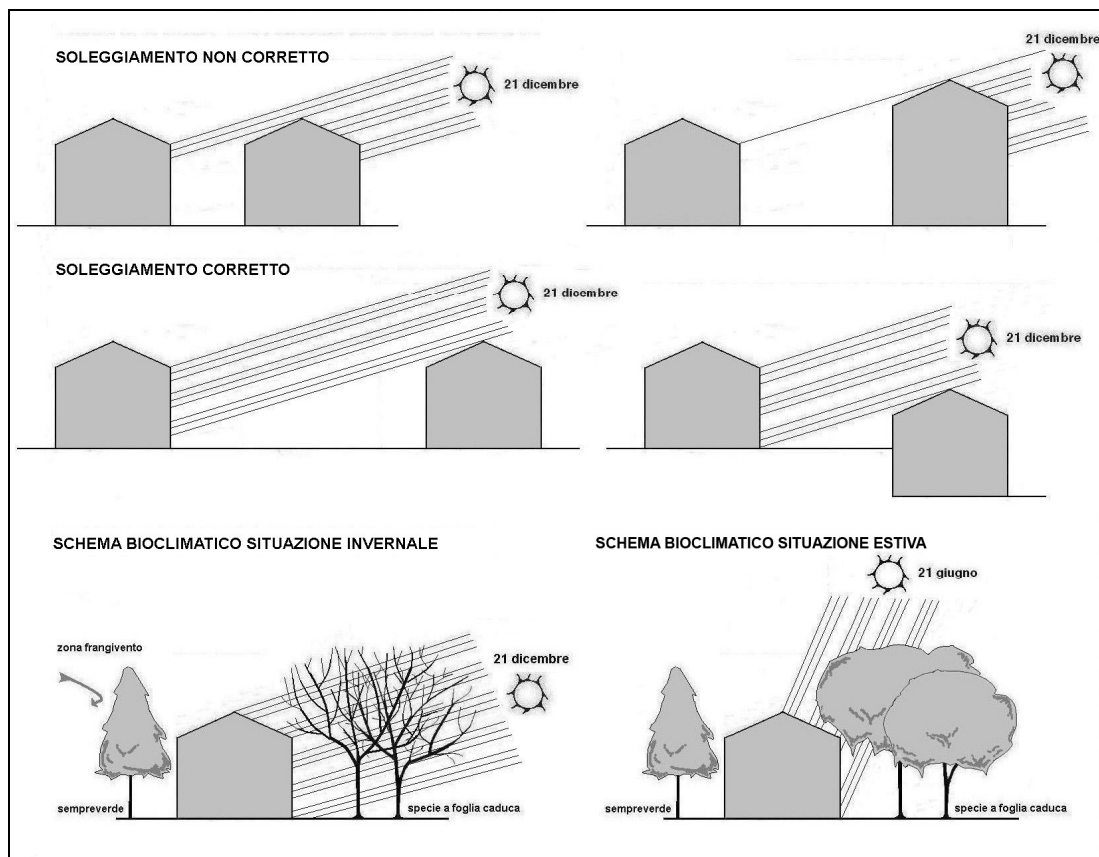
Nuova edificazione – Residenza – Soleggiamento degli edifici
