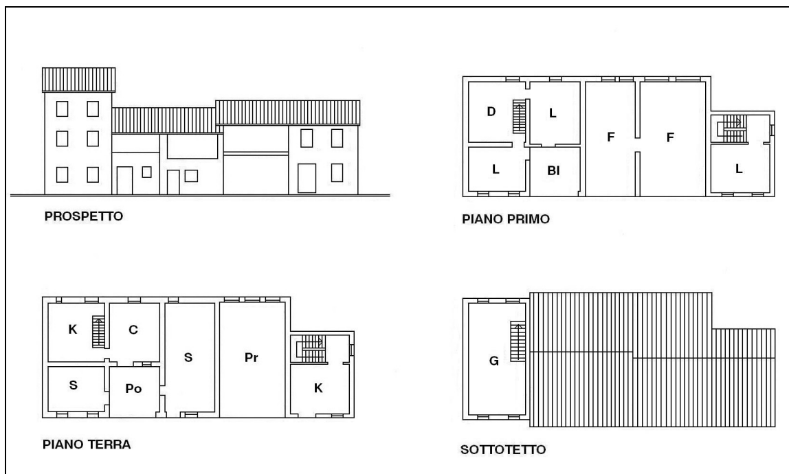
Tipologia ad elementi giustapposti
