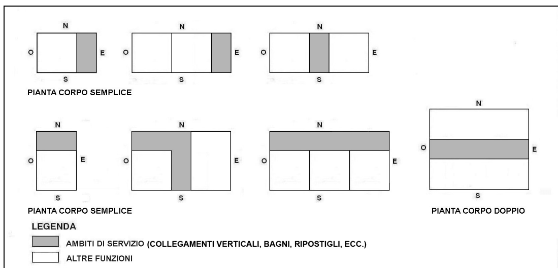
Nuova edificazione – Residenza – Aggregazioni tipologiche con localizzazione ambiti di servizio
