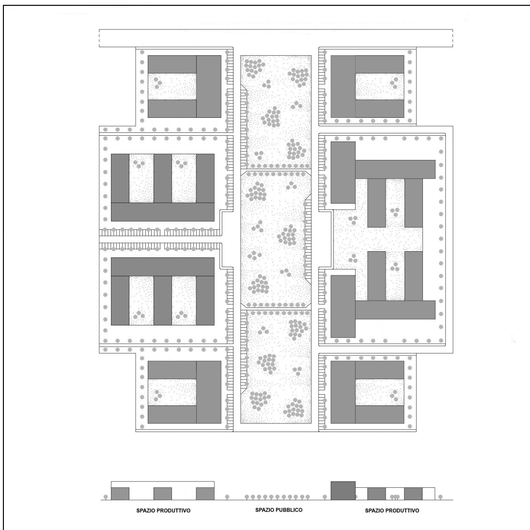
Ambiti produttivi di trasformazione – Schema esemplificativo
