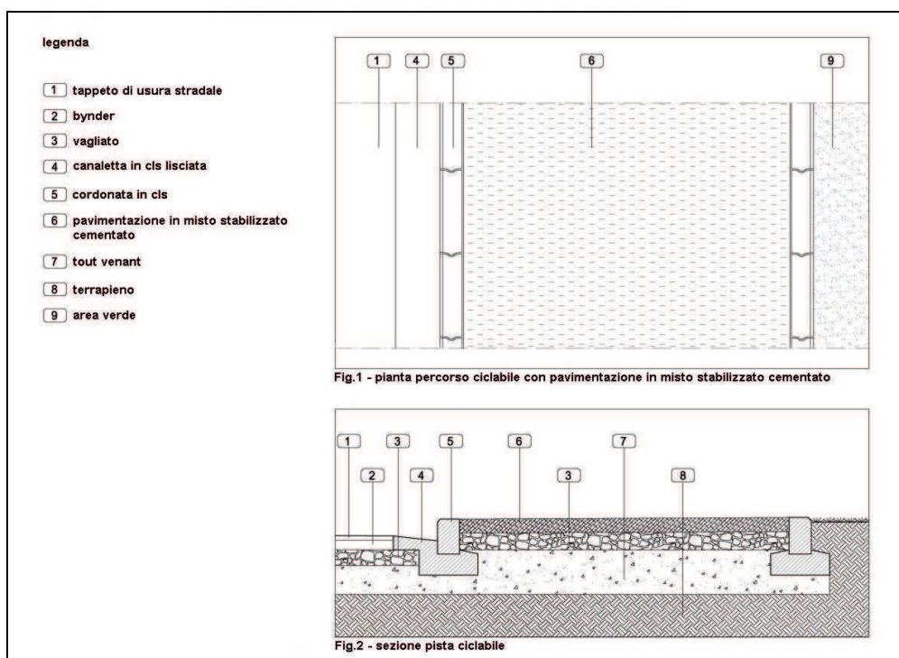
Schema percorso ciclopedonale con pavimentazione in misto stabilizzato cementato
