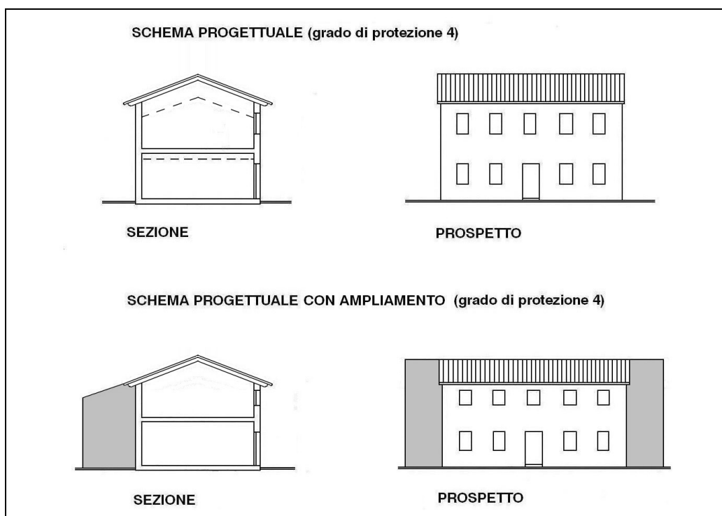
Esemplificazione interventi di recupero dell'esistente con grado di protezione 4
