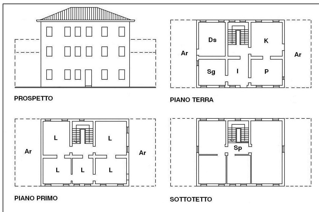
Tipologia con copertura a padiglione
