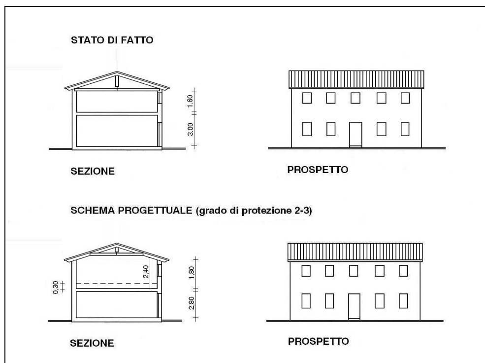
Esemplificazione interventi di recupero dell'esistente con grado di protezione 2-3
