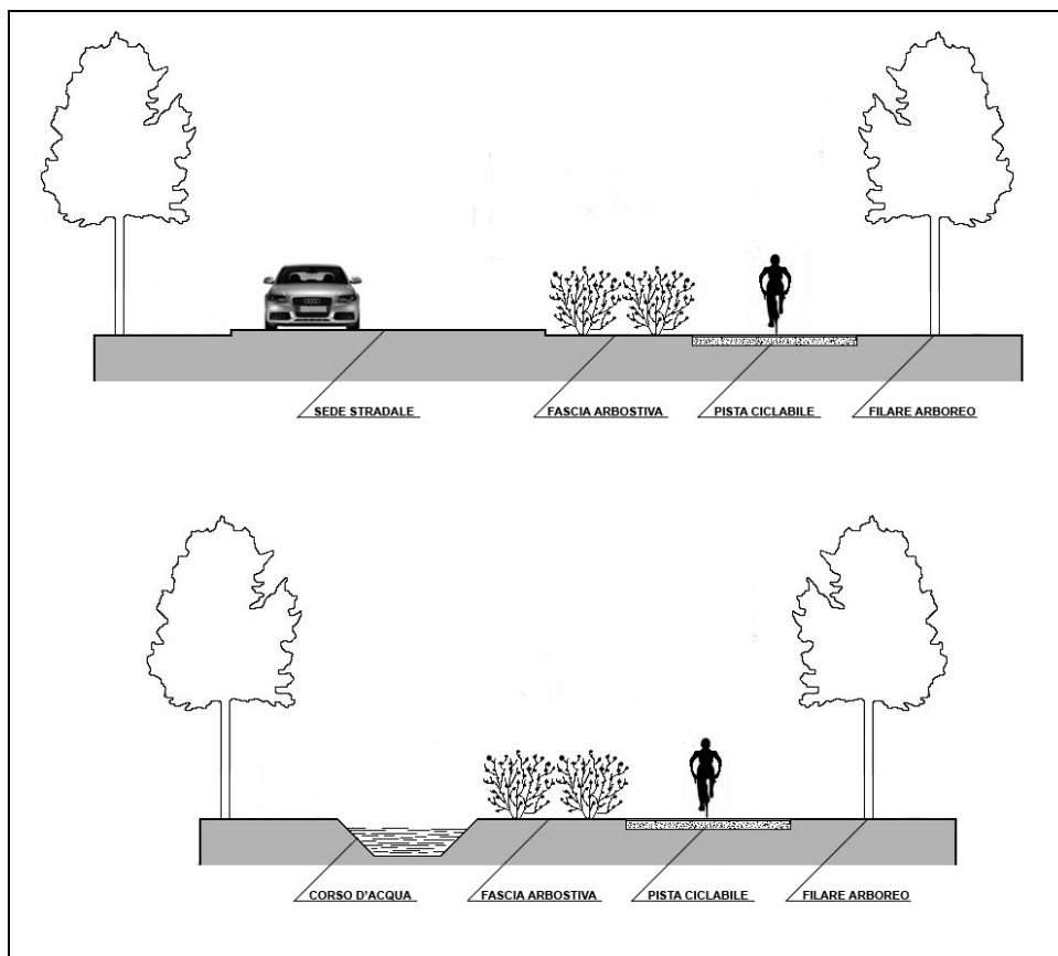
Schemi tipo percorsi naturalistici ciclopedonali
