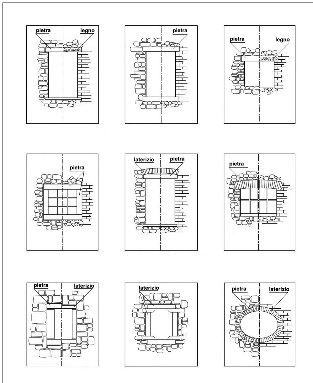
D.8.1 – Finestre - Modelli tipologici edilizia tradizionale
