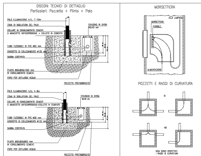
Figura 43. Schemi di massima, sostegni, pozzetti e giunzioni.
